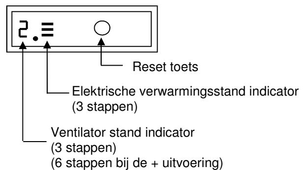
Display uitlezing LU toestel elektrisch verwarmd
