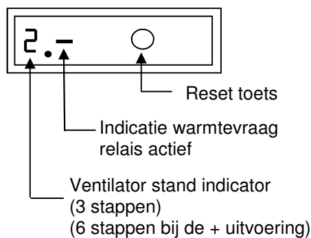
Display uitlezing LU toestel cv water verwarmd
