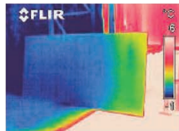
Luchtdeur ingeschakeld
